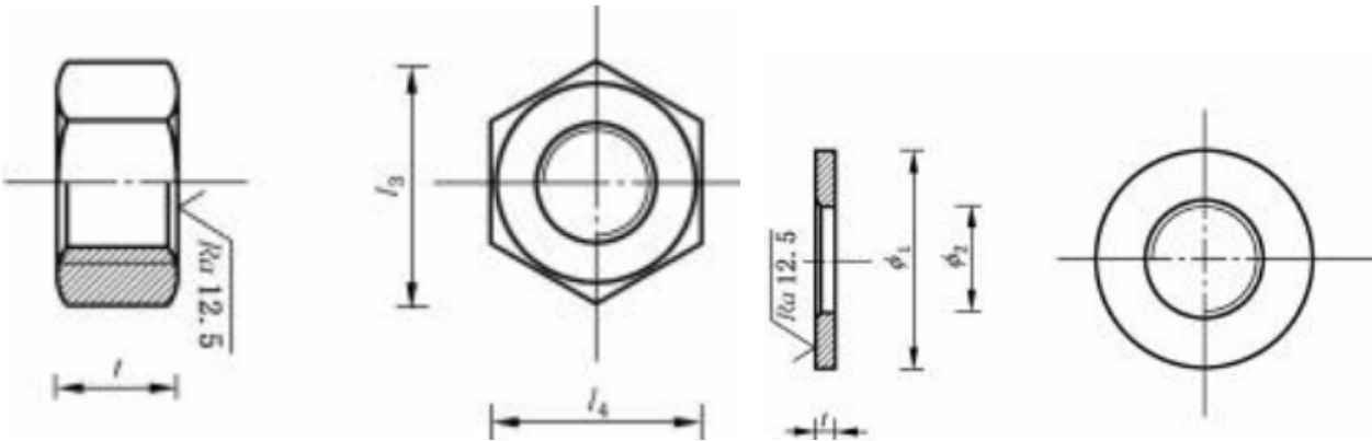
b) 螺母J II -3
