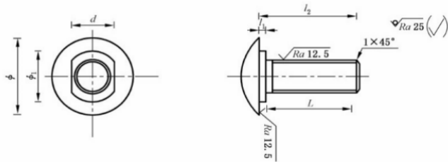
a) 拼接螺栓 J I -1、J I -2
